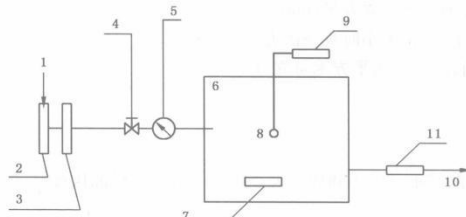
1—空气进气口；2—空气过滤器；3—空气温湿度调节系统；4—空气气流调节器； 5—空气流量调节器；6—密封舱；7—气流速度和空气循环的控制装置；8—温度和 湿度传感器；9—温度和湿度的监测系统；10—排气口；11—空气取样的集气管
